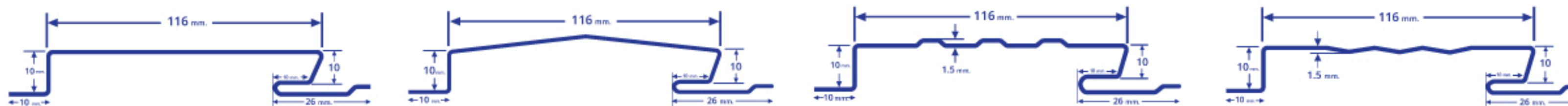
แบบติดชิด-ฝ้า
