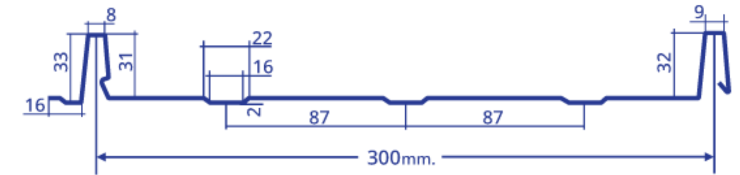
ลาย3ตะเข็บ
