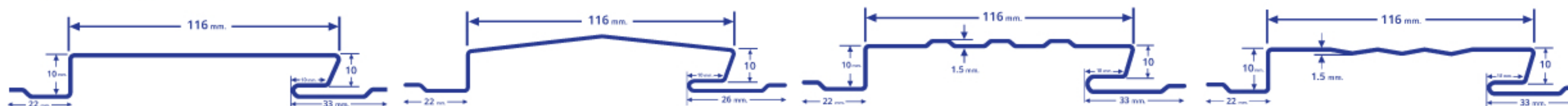
แบบเว้นร่อง-ผนัง
